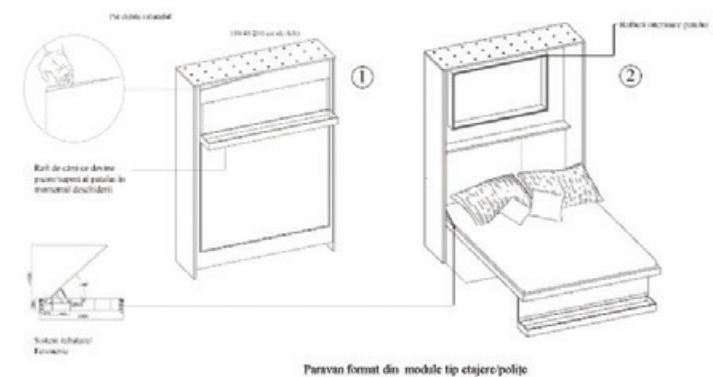
Paravan format din module tip etajere/polițe
