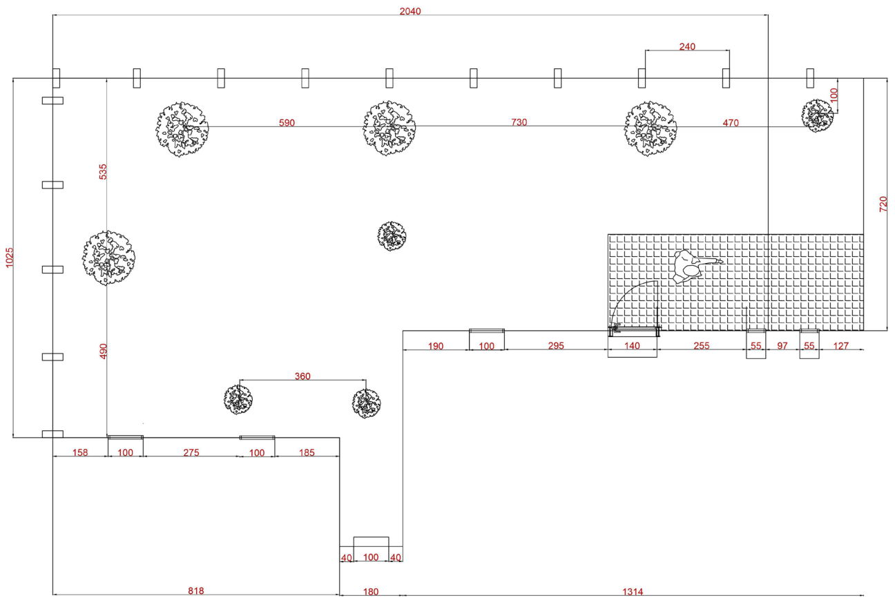
Relevu pentru amenajarea exterioară
